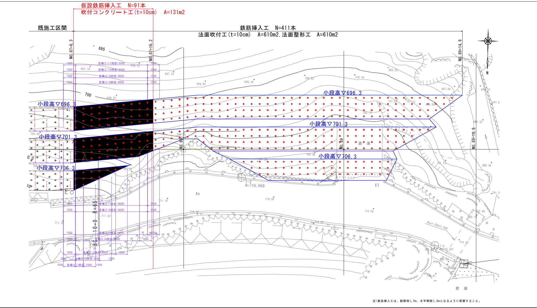
平面図
